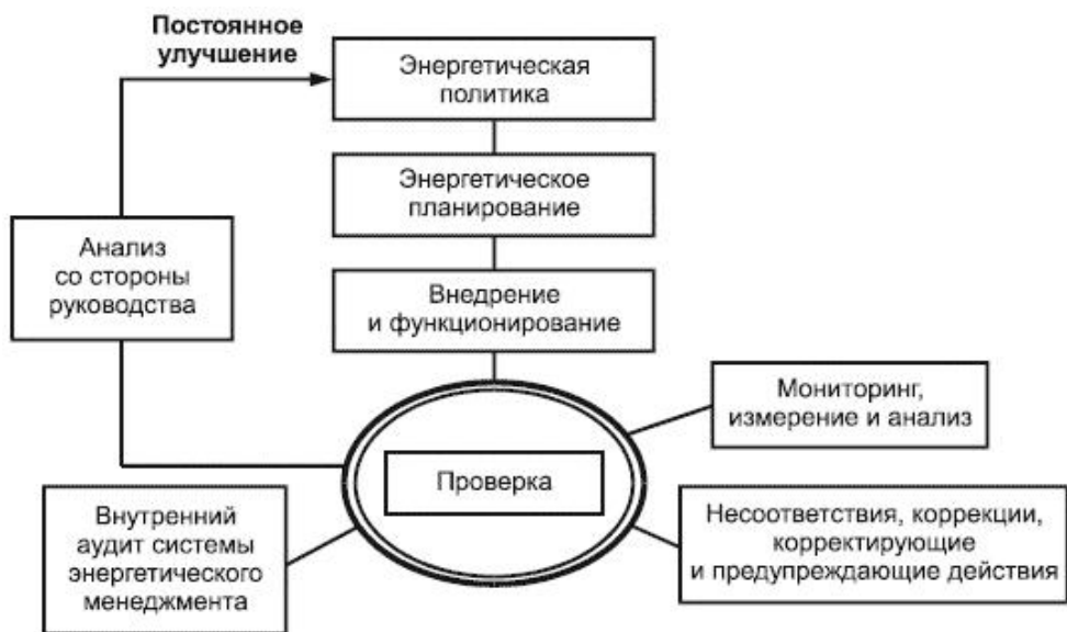
Рисунок 1 - Модель системы энергетического менеджмента для настоящего стандарта
